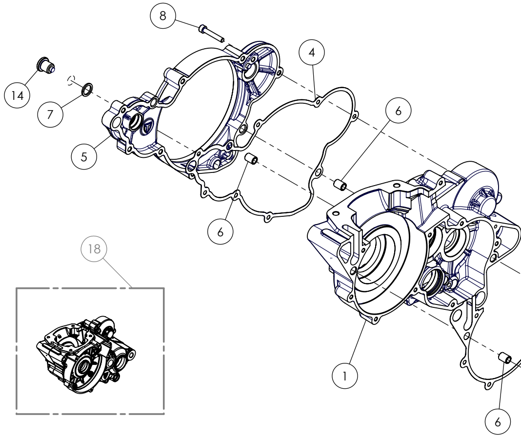
Graphic Engine Longer Bolts - Gráfico Longitud Tornillos
